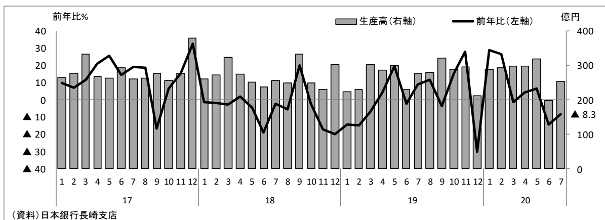
【機械・重電生産高】
